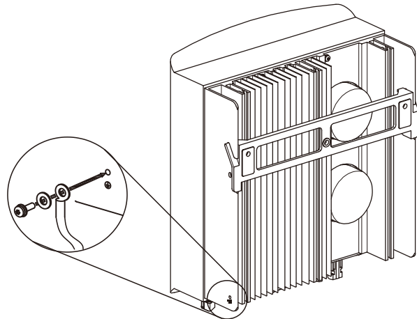
Ilustración 4.19 Conectar el conductor externo de tierra
